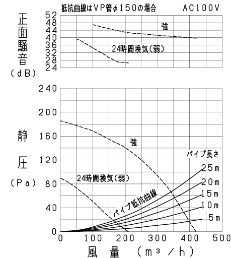
VD-20ZLC 13 -IN/P-Q・騒音特性
